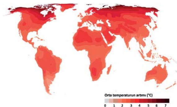
B. 2050-ci ilə qədər global temperatur artımı
