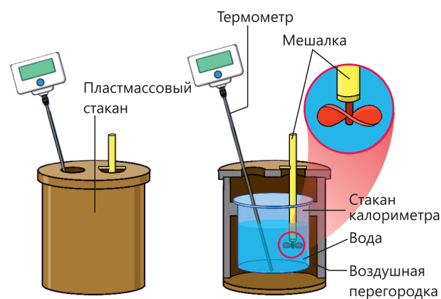
Рис. 6.1. Лабораторный калориметр.
