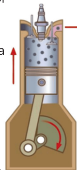
Рис. 6.9. Цилиндр двигателя внутреннего сгорания.
