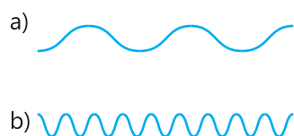
Рис. 4.9. Камертоны с разной частотой колебания издают звуки разной тональности.
