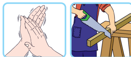
Рис. 5.7. Увеличение внутренней энергии за счет совершения работы.
