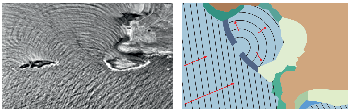
Рис. 4.14. Дифракция волн, распространяющихся на поверхности воды.
