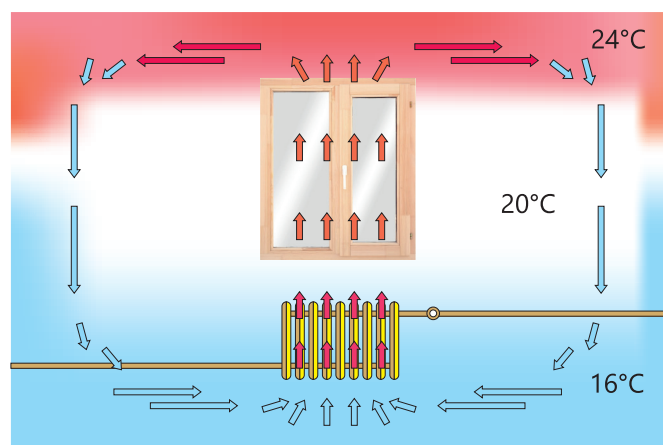
Рис. 5.10. Конвекция в газе.
