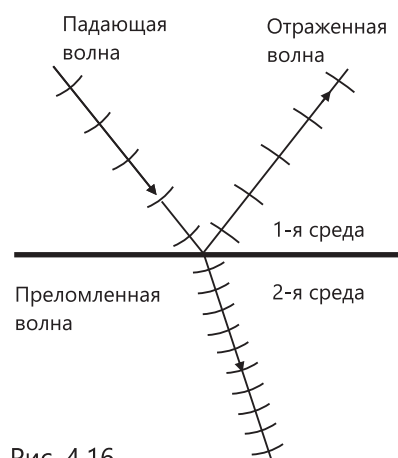
Рис. 4.16. Отражения и преломления волн.
