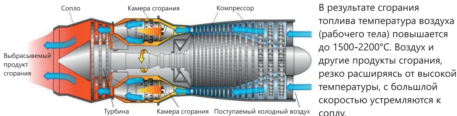
Рис. 6.12. Схема строения и принципа работы газового (воздушного) реактивного двигателя.
