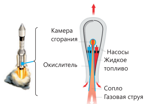
Рис. 6.13. Схема принципа работы ракетного двигателя.
