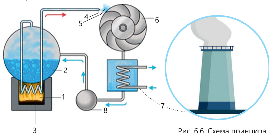
Рис. 6.6. Схема принципа работы парового двигателя.
