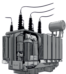
Трансформатор
