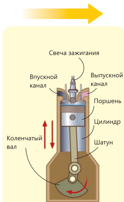
Рис. 6.9. Цилиндр двигателя внутреннего сгорания.
