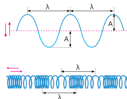
Рис. 4.4. Длина волны в поперечных и продольных волнах.
