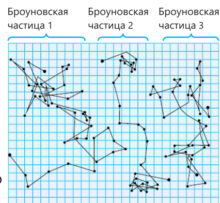
Рис. 5.1. Траектория движения броуновской частицы.
