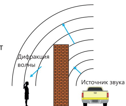
Рис. 4.15. Дифракция звука.
