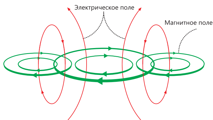
Рис. 4.17. Электромагнитное поле.
