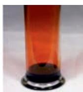
пары брома
