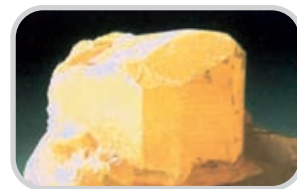
При комнатной температуре устойчивой формой серы является ромбическая сера.
