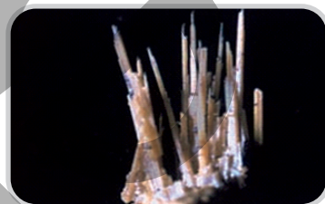
Rombik kükürd 96^\circ\text{C} -dən yuxarı temperaturda tədricən qızdırıldıqda onun kristal quruluşu dəyişir. Nəticədə molekullar fərqli şəkildə düzülərək iynə formalı monoklinik kükürd kristalları əmələ gətirir.
