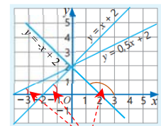
Угол, образованный прямой с положительным направлением оси Ox
