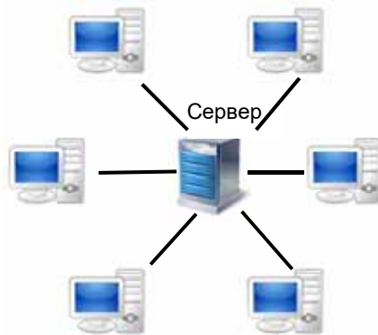
Сеть "клиент-сервер"
