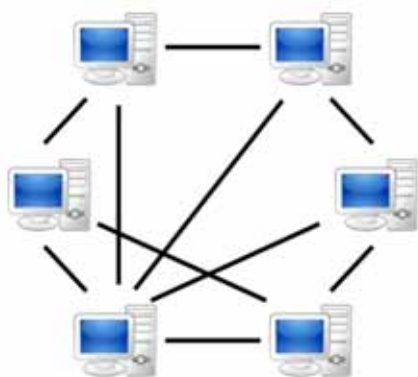
Одноранговая сеть
