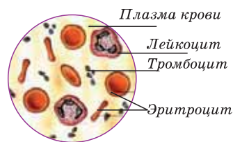
Состав крови
