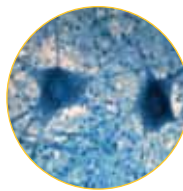
Нервная ткань
