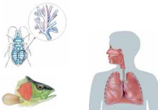
Дыхательная система
