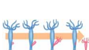
Гидра
