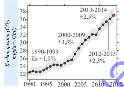
Atmosferdə karbon qazının miqdarının dəyişməsi (1 Giqaton (Gt) = 10^9 t)
