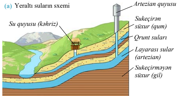
(a) Yeraltı suların sxemi
