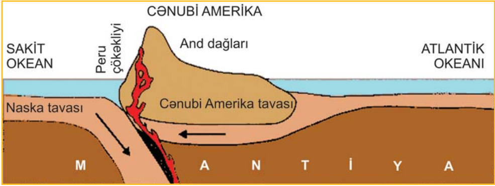
Materik və okean tavalarnın toqquşma sərhədi
