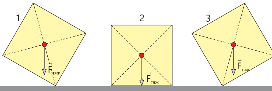
Рис. 7. Опрокинется тело под действием силы или нет, зависит от того, где находится – линия действия силы тяжести внутри или снаружи площади опоры.
