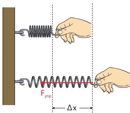
Рис. 2. В растянутой пружине возникает сила упругости.
