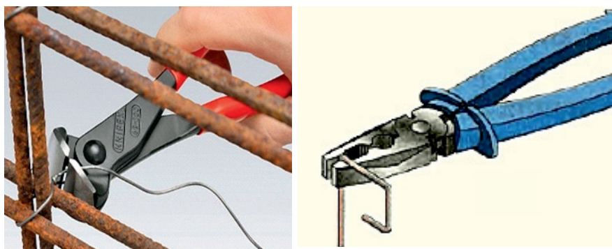
Рис. 1. Плоскогубцы, используемые для перекусывания и сгибания проволоки.
