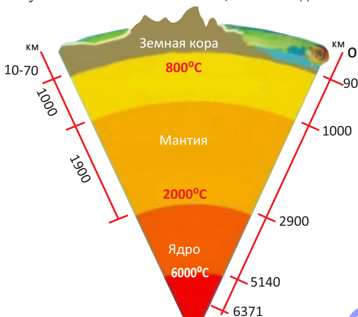
Внутреннее строение Земли
