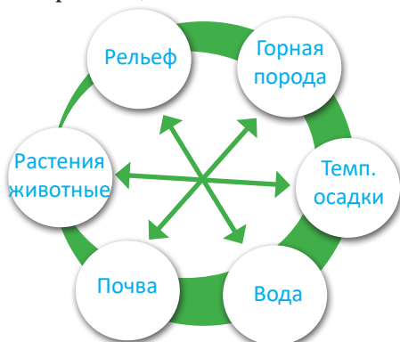
Взаимодействие природных компонентов
