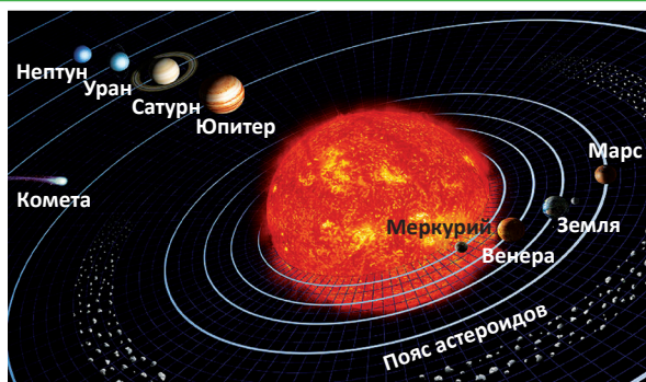
Солнечная система
