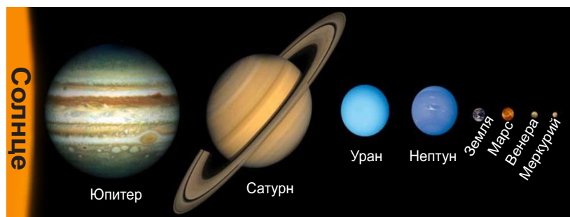
Сравнение размеров планет
