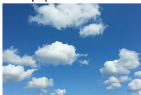
Парообразное состояние воды
