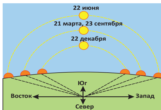
Изменение положения восхода и захода Солнца над горизонтом, являющегося причиной изменения продолжительности дня и ночи.
