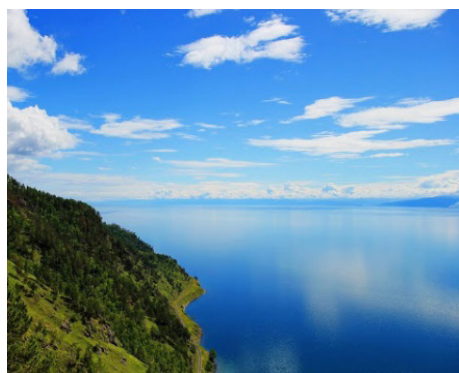
В Байкале сконцентрировано 20% мировых запасов пресной воды
