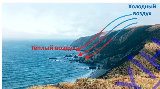
Ветра в прибрежной зоне
