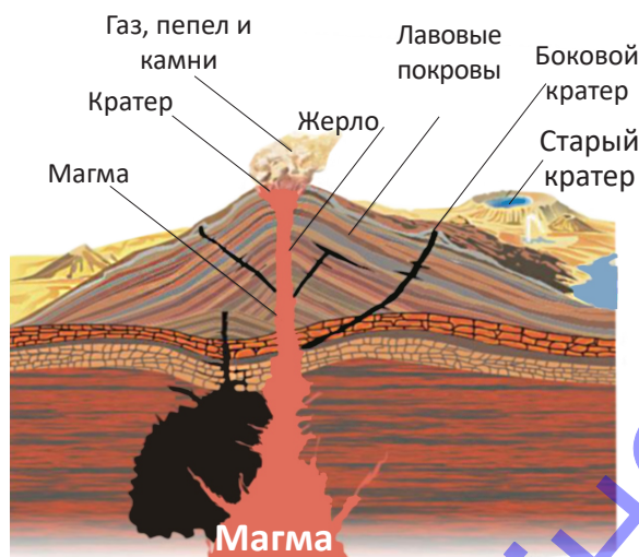
Вулкан в разрезе
