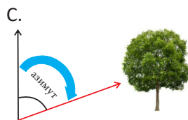
Азимут и его определение
