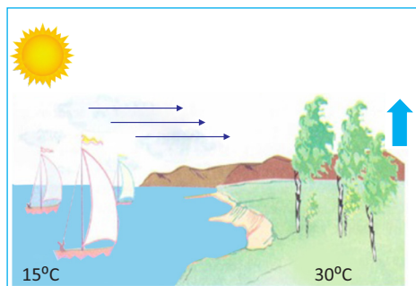
Движение воздуха между сушей и водой
