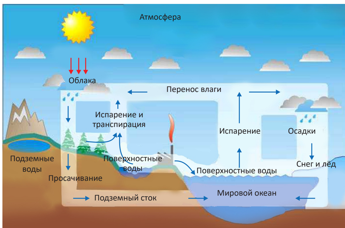
Круговорот воды в природе
