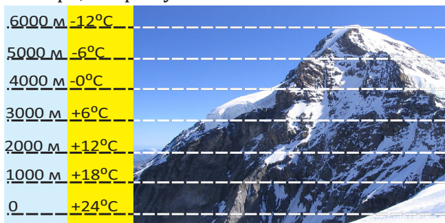
Уменьшение температуры с высотой
