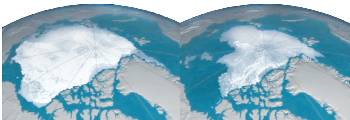
Площади ледников в Арктике сокращаются
