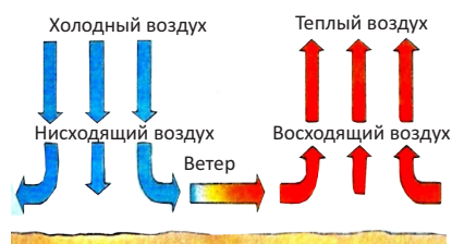
Потоки, образующиеся в результате нагрева и охлаждения воздуха
