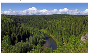
Хвойный лес (тайга)
