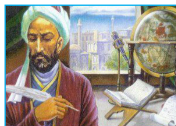
Н.Туси
