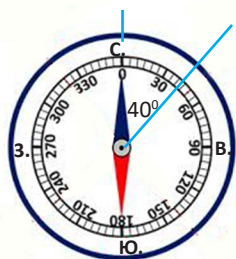
Азимут и его определение
