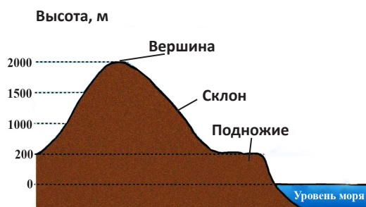
Основные элементы горы
