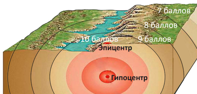
Очаг землетрясения и распространение сейсмических волн
