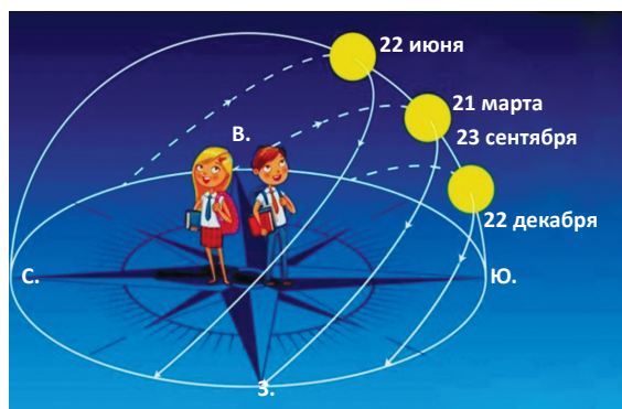
Изменение высоты Солнца над горизонтом в течение года
