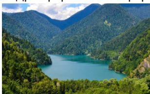
Жидкое состояние воды
