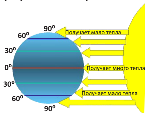
Нагрев земной поверхности зависит от угла падения солнечных лучей
