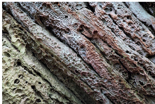
Результаты химического выветривания
