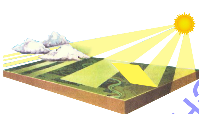
Нагрев земной поверхности зависит от угла падения солнечных лучей
