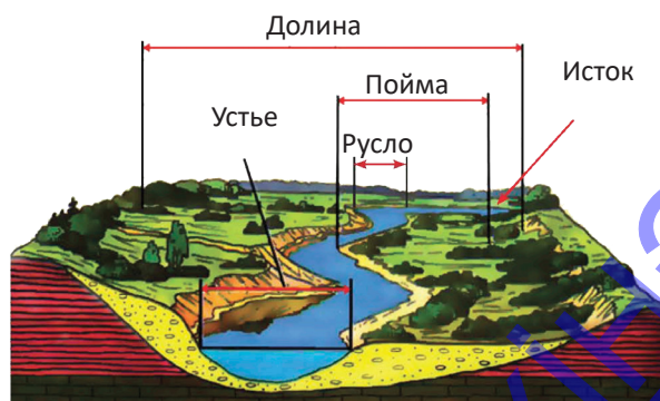
Речная долина и ее элементы
