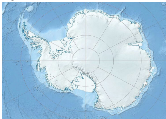
Ледяной покров Антарктиды
