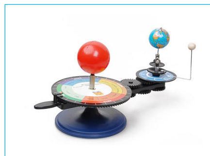
Теллурий
