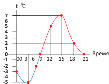
График среднесуточной температуры
