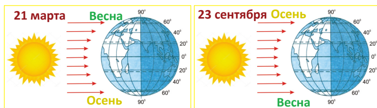
Состояние равного нагрева и освещенности поверхности Земли Солнцем.
