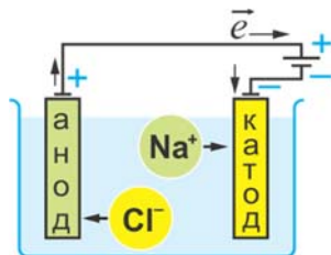
Электролиз расплава NaCl (схема)
