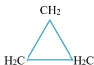
циклопропан \text{C}_3\text{H}_6
