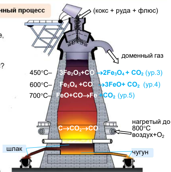
(a) Доменная печь
