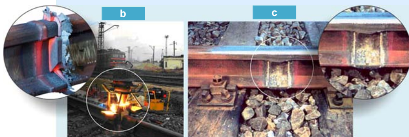
b – Термитная сварка рельсов способом алюминотермии; c – рельс после термитной сварки.
