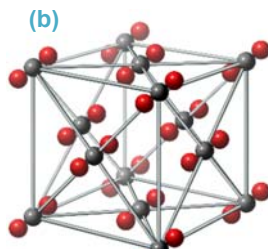
Диоксид углерода
