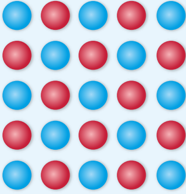
Homogen qarışıq
