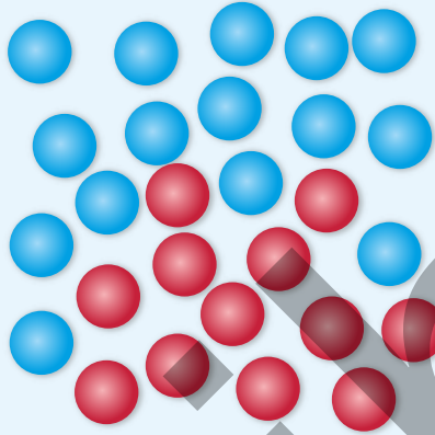
Heterogen qarışıq
