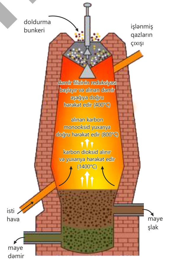
Domna sobası
