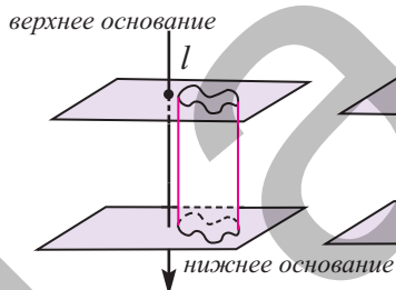
Прямой цилиндр
