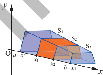
различные сечения
