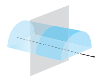
одинаковые сечения
