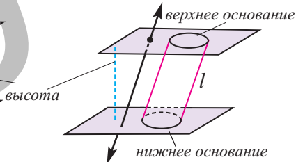
Наклонный цилиндр
