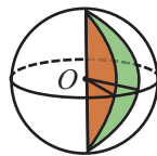
долька шара
