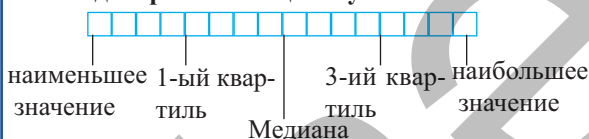
Схематическое представление диаграммы “ящик с усами”
