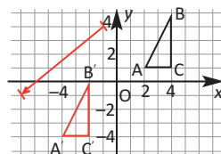
Paralel köçürmə vektoru: \langle -6; -5 \rangle
