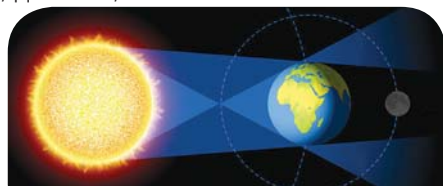
Лунное затмение
