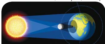
Солнечное затмение
