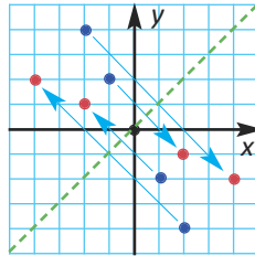
y = x oxuna nəzərən əksətmə nümunələri
