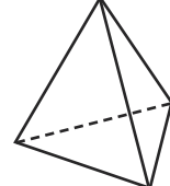
Üçbucaqlı piramida
