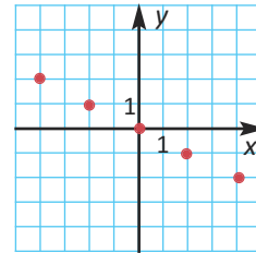
Tərs funksiyanın qrafiki
