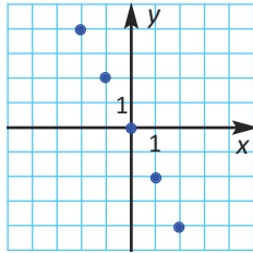
Verilən funksiyanın qrafiki
