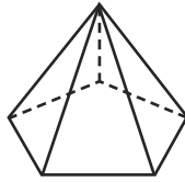
Beşbucaqlı piramida
