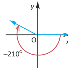
mənfi bucaq
