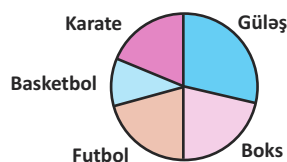
Dairəvi diaqram
