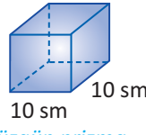
düzgün prizma
