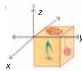
180^\circ dönmə
