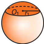
kürə seqmenti
