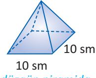
düzgün piramida
