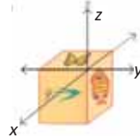
270^\circ dönmə
