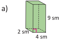
düzbucaqlı paralelepiped
