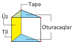
Üçbucaqlı prizma
