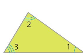
Üçbucağın daxili bucaqları
