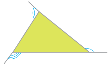
Üçbucağın xarici bucaqları
