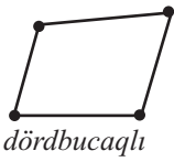
dördbucaqlı
