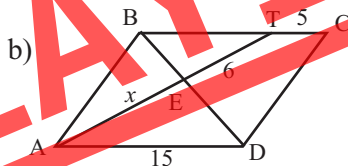
ABCD paraleloqram
