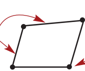
dördbucaqlı
