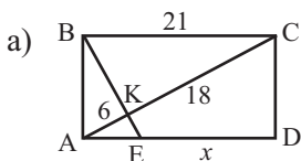
ABCD düzbucaqlı
