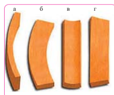
Рис. 3. Виды коробления досок: а, б – продольное; в – поперечное; г – винтовое
