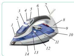
Рис. 1. Электрический утюг: 1 – разбрызгиватель воды; 2 – крышка, закрывающая отверстие для заливки воды; 3 – рычажок, регулирующий постоянную подачу пара; 4 – кнопка для разбрызгивания пара; 5 – кнопка для дополнительной подачи пара; 6 – ручка утюга; 7 – вставка для защиты электрического шнура от перегибов; 8 – основа утюга; 9 – сигнальная лампочка; 10 – емкость для воды; 11 – рукоятка регулятора температуры глажки; 12 – включение режима самоочистки; 13 – отметка, показывающая уровень воды в резервуаре; 14 – подошва утюга
