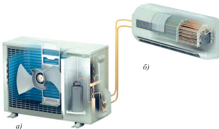
Рис. 2. Кондиционер сплит-система
