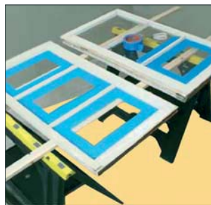
Рис. 7. Защита стекла скотчем
