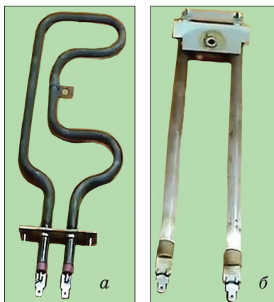
Рис. 4. Грили: а) ТЭН-овый; б) кварцевый
