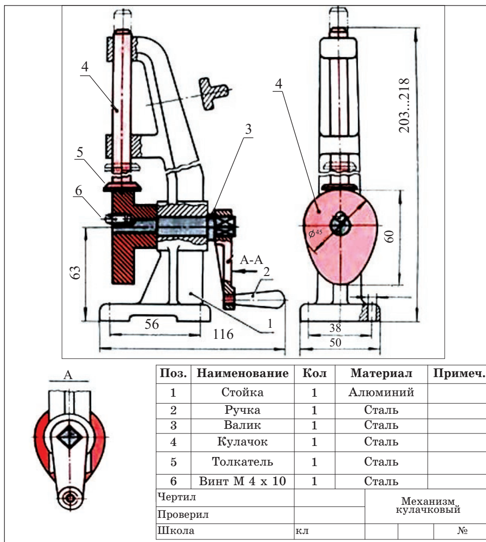
Рис. 2. Сборочный чертеж кулачкового механизма
