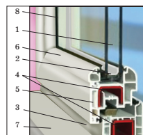
Рис. 2. Отрезок пластикового окна:
