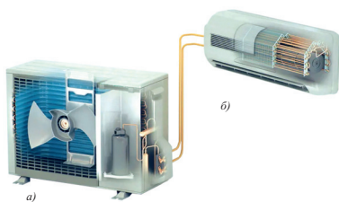
Рис. 2. Кондиционер сплит-система
