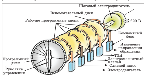
Рис. 4. Схема связи редуктора с различными компонентами стиральной машины
