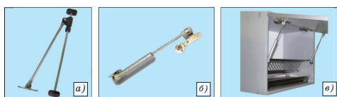
Рис. 8. Мебельные кронштейны: а – пластиковый; б – с газовыми стойками; в – соединение деталей
