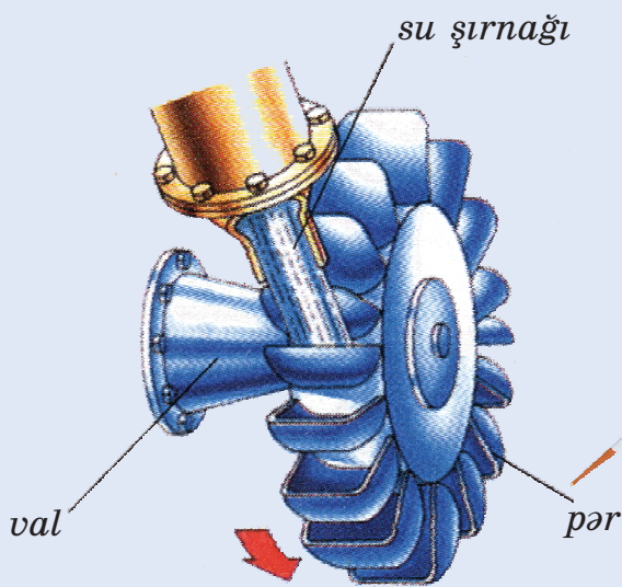
Çalovlu su turbini
