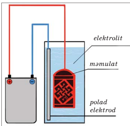
Şəkil 7. Məmulatın aşınma sxemi
