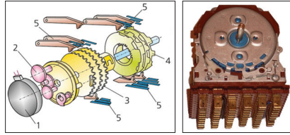
Şəkil 3. Elektromexaniki taymerin quruluşu: 1 - addımlı elektrik mühərriki; 2 - ötürücü dişli çarxlar; 3 və 4 - yumrucuqlar pəketi; 5 - sürüşən kontaktlar
