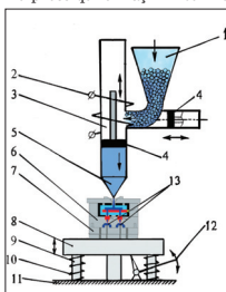
Şəkil 3. Tökmə maşının sxemi
