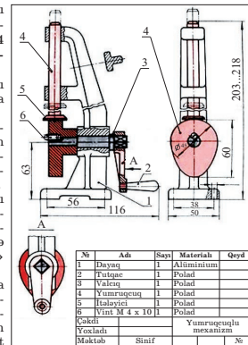
Şəkil 2. Yumruqcuqlu mexanizmin yığma certyoju
