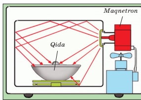
Şəkil 3. İşçi kameranın divarlarından mikro dalğaların əks olunması
