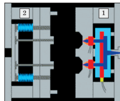
Şəkil 5. Press-qalib
