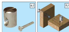
Şəkil 3. Vintli bərkitmə: a) vintlər; b) detalların birləşməsi
