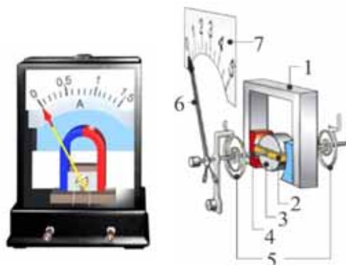
(e) Амперметр и его устройство
