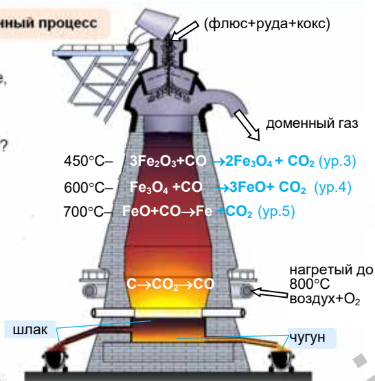
(а) Доменная печь
