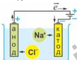
Электролиз расплава NaCl (схема)
