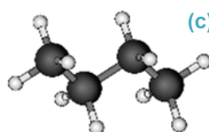
Шаростержневые и шаровые модели молекул метана (a), этана (b) и бутана (c)
