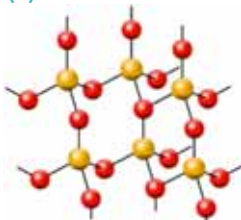
Диоксид кремния
