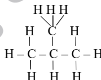
изобутан \text{C}_4\text{H}_{10}
