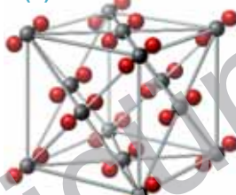
Диоксид углерода
